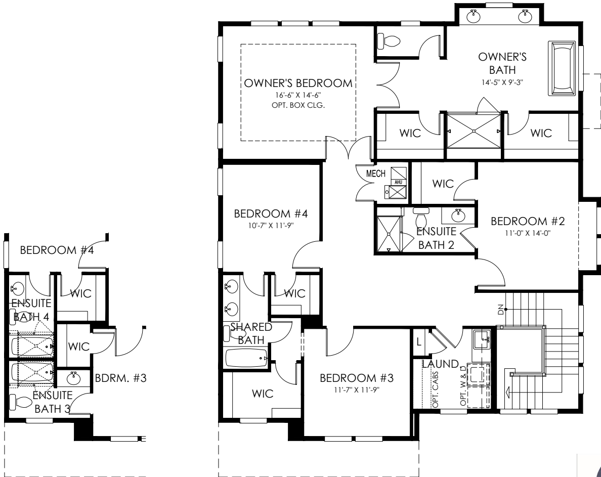
OPT. ENSUITE BATH 3 & 4
